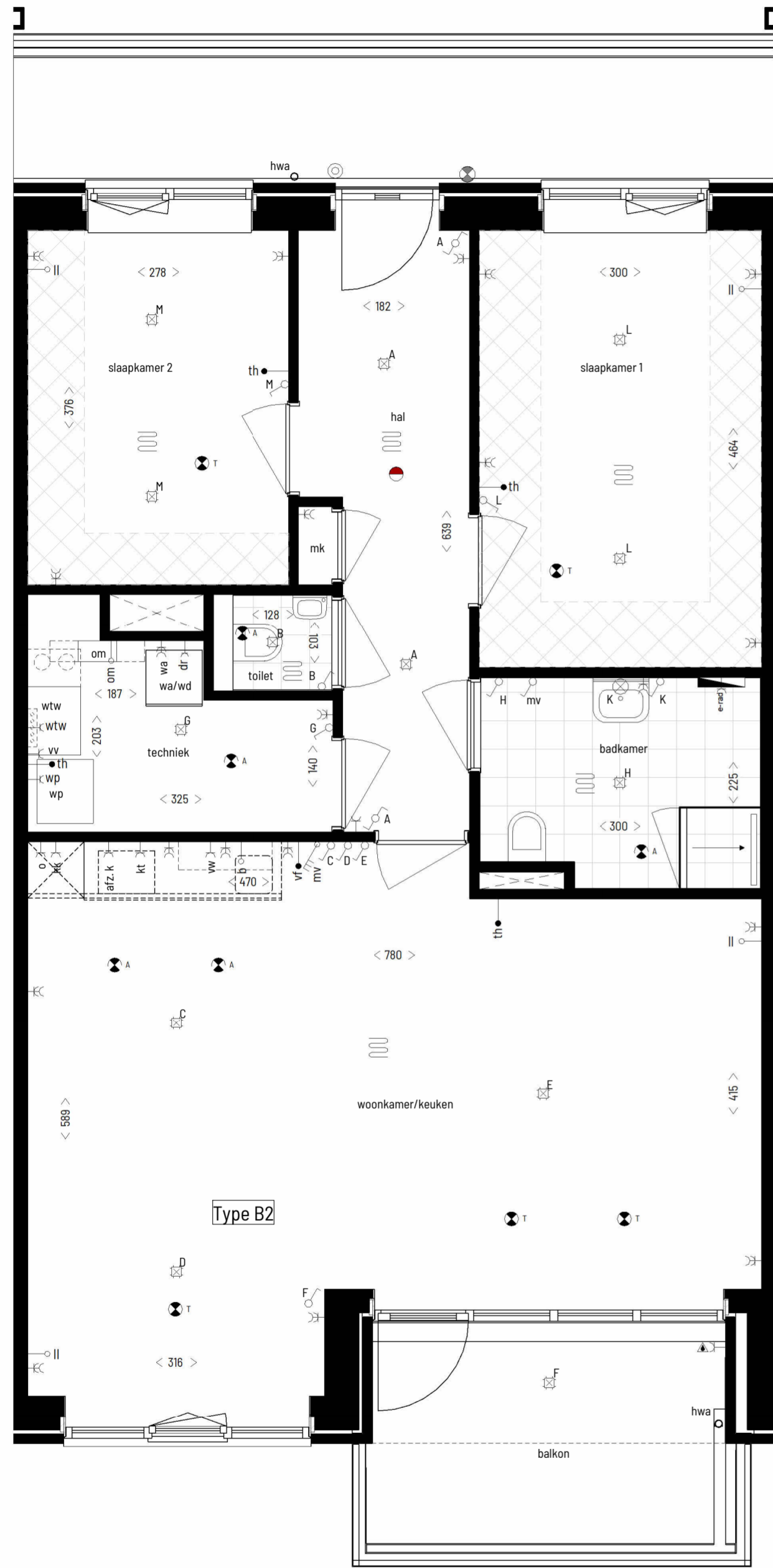
eerste verdieping
